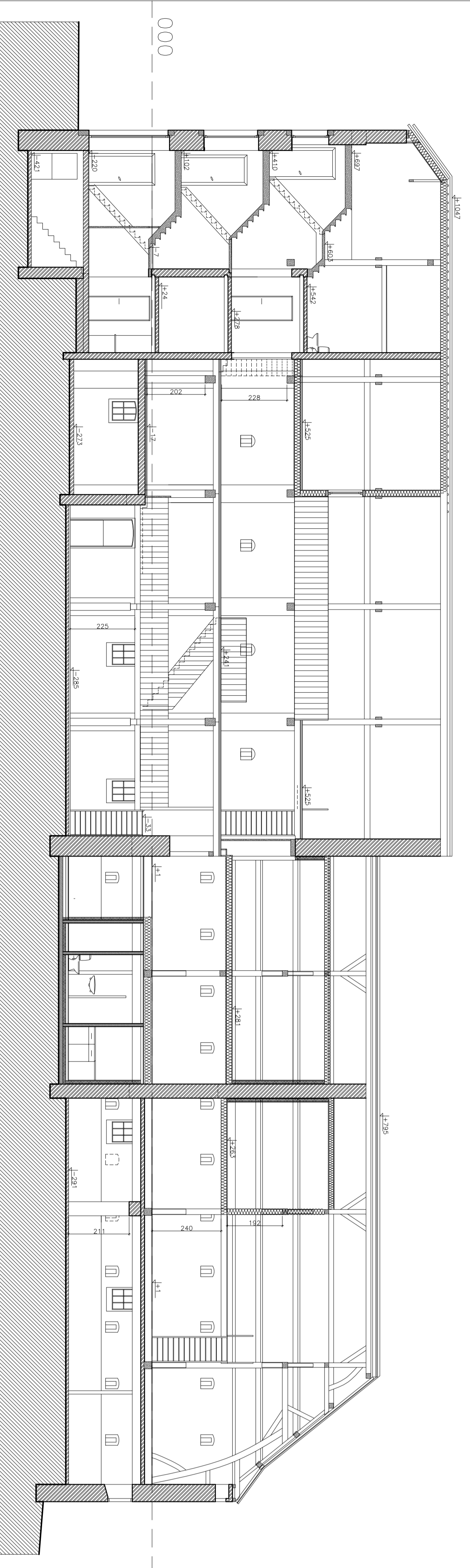
FAÇADE SUD-OUEST
