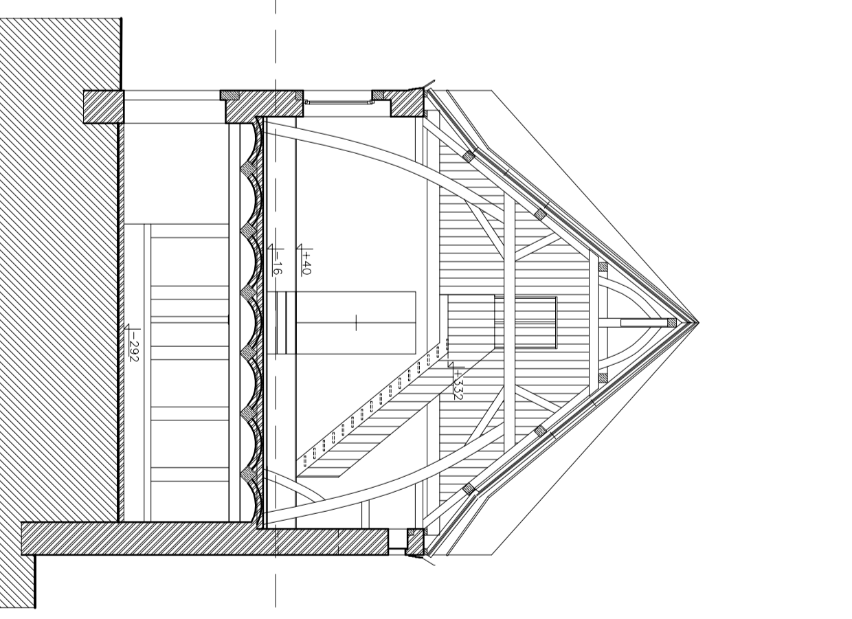
COUPE FF AILE NORD
